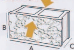
Bloque 2 caras Split
